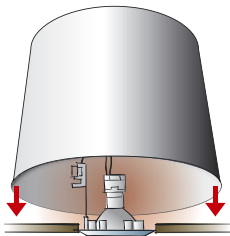
Inbyggd halogenlampa ska monteras med värmeskydd
